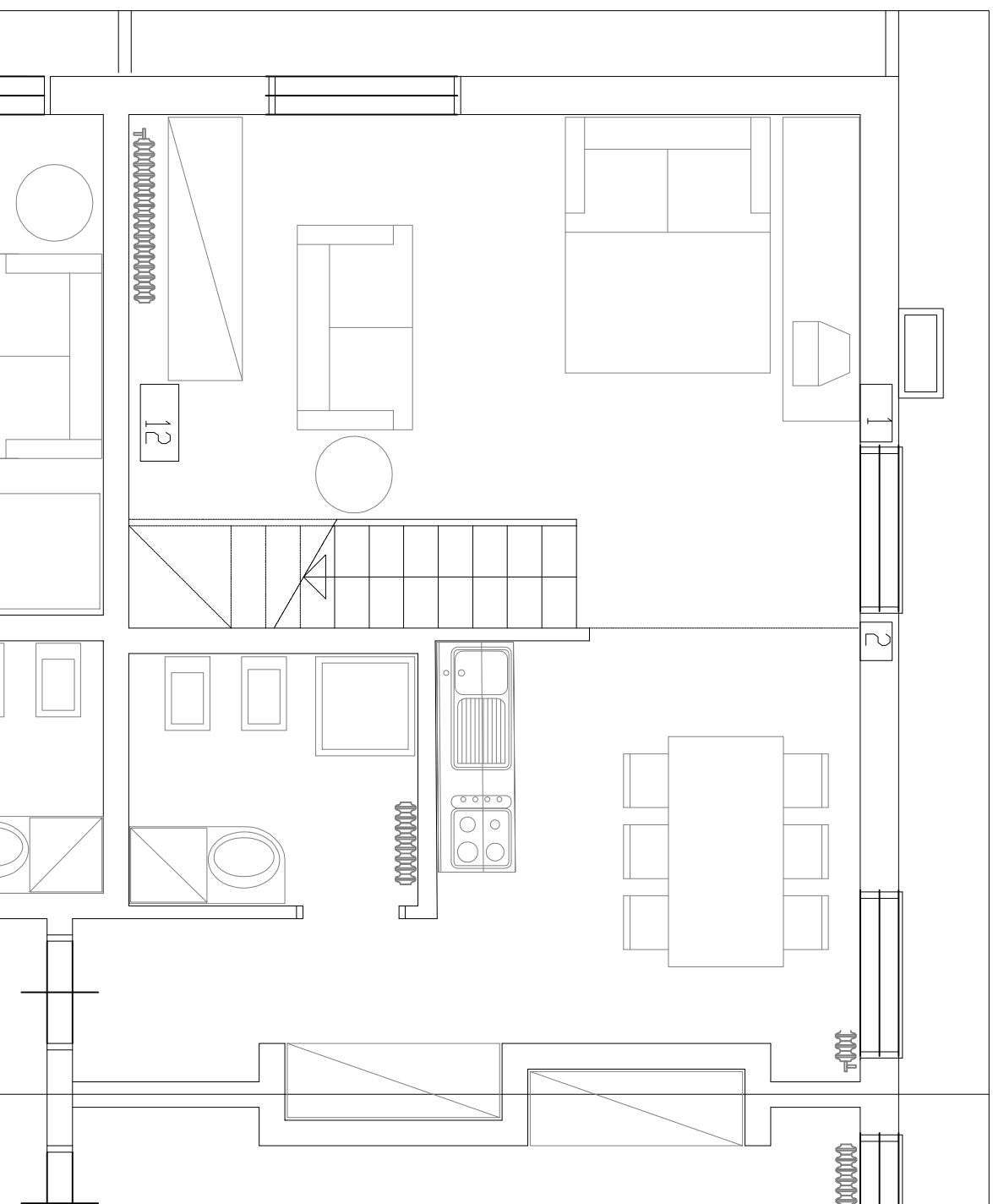
PIANO +1 APPARTAMENTO 165
