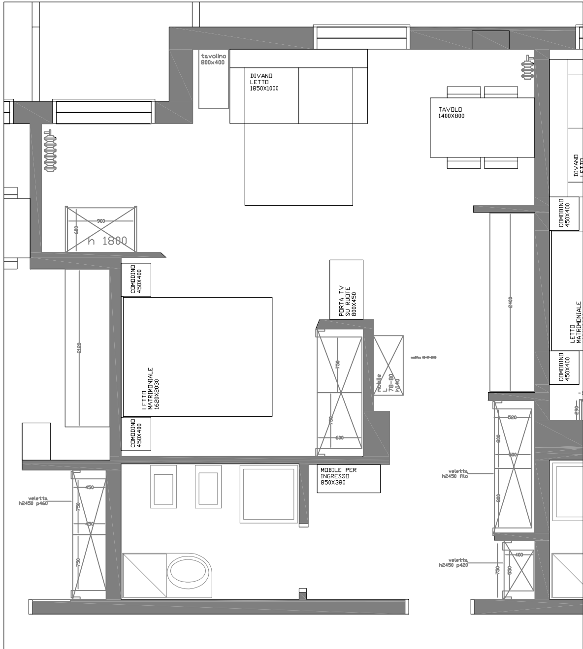
PIANO -2 APPARTAMENTO 140
